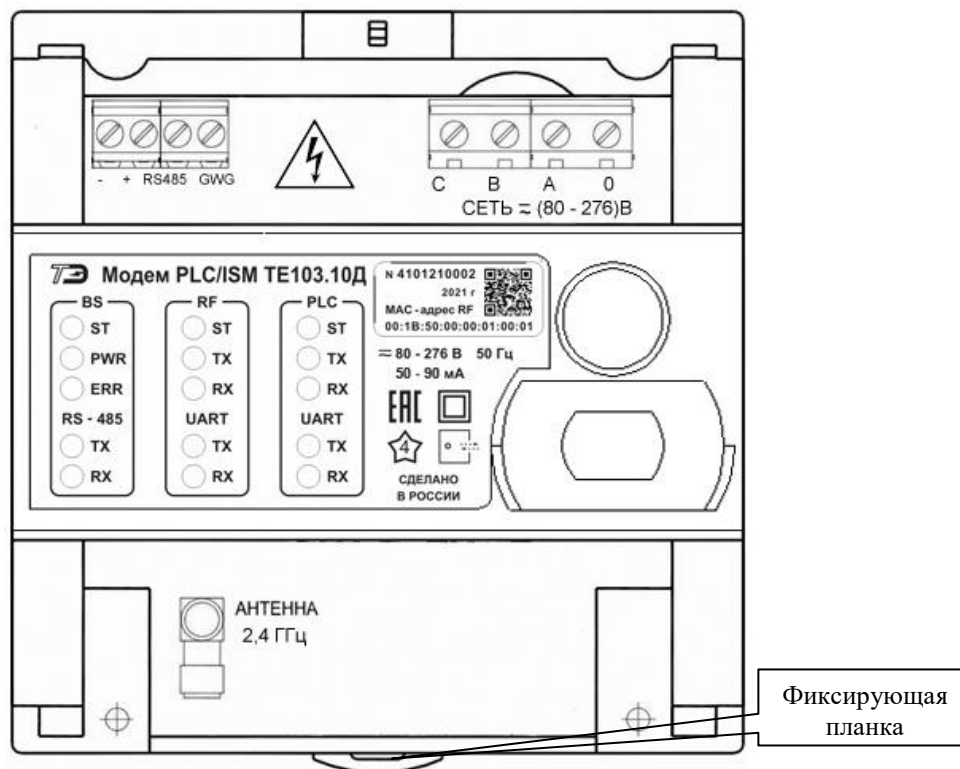
Рисунок А.4 - Расположение элементов подключения под защитными крышками модемов TE103.10Д, TE103.01Д, TE103.02Д
