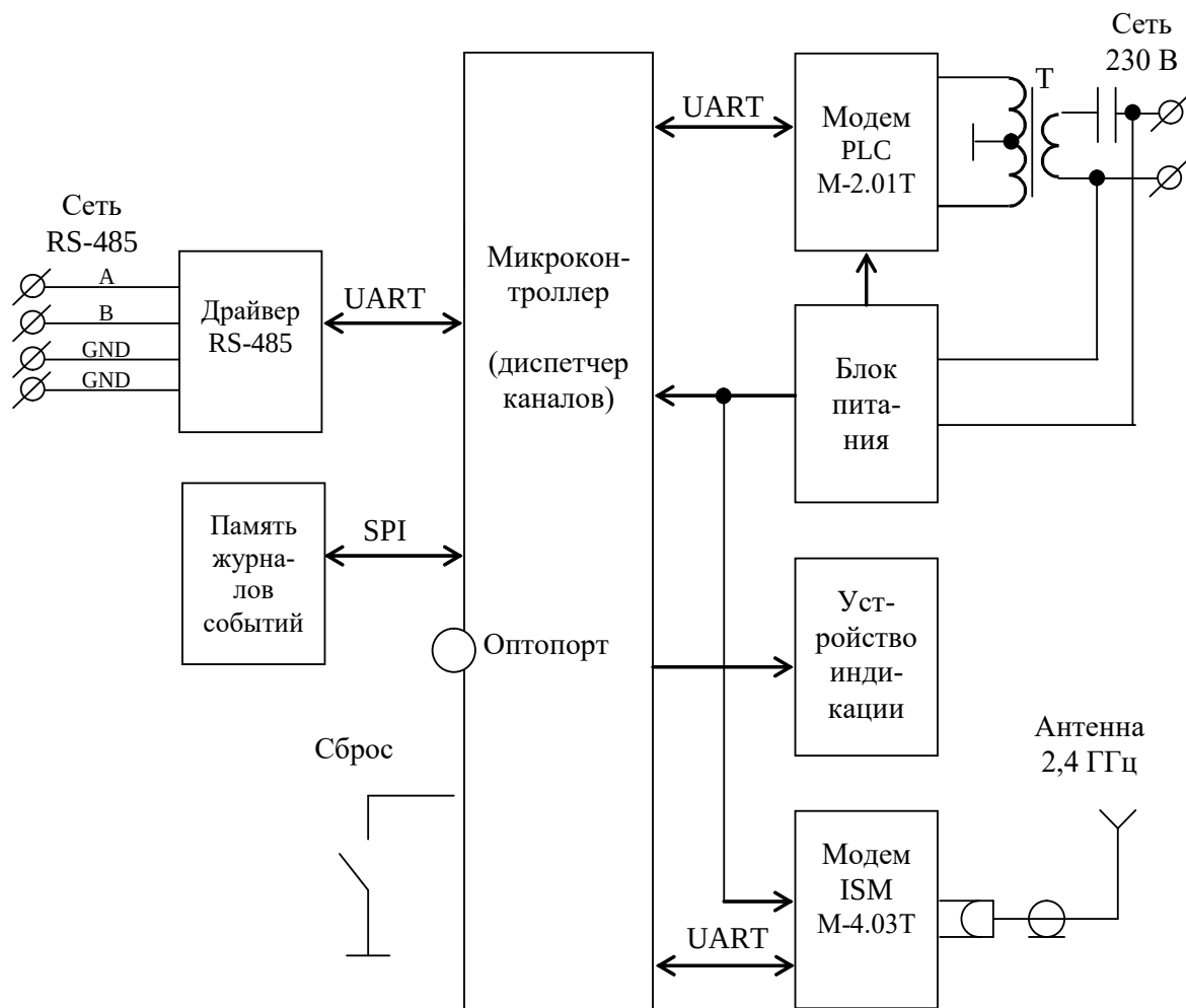
сунок 1 – Структурная схема модема
