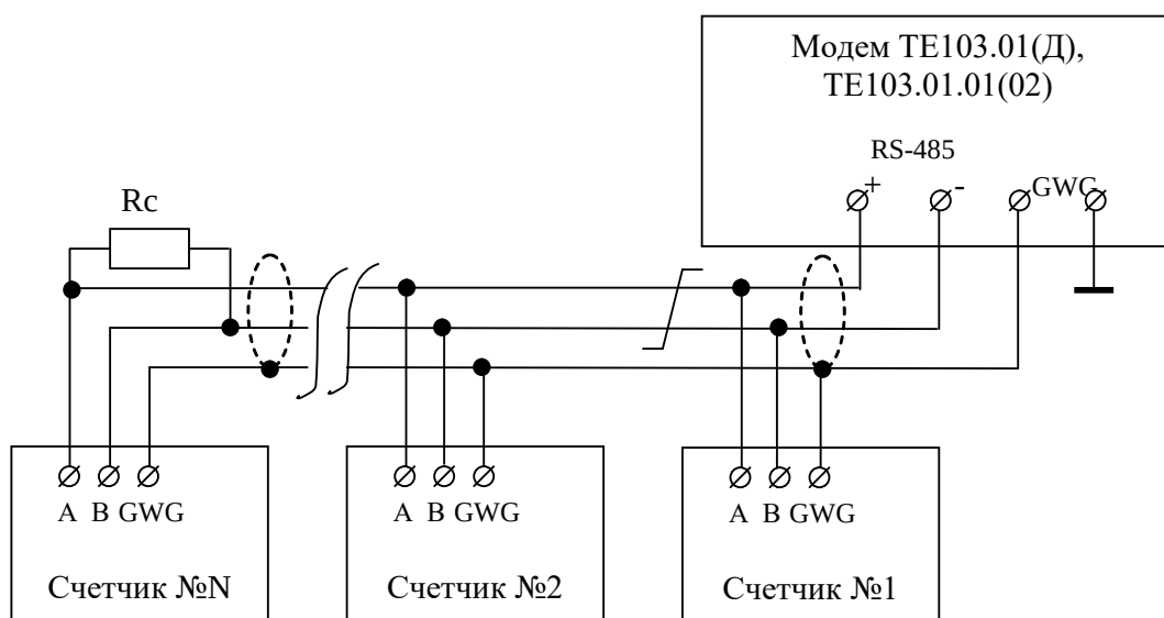
Рисунок Б.5 - Схема подключения встроенной удаленной станции TE103.01.01A к компьютеру и к электрической сети
