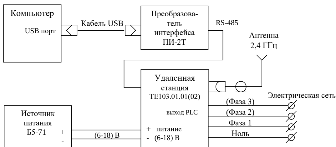
Рисунок Б.3 - Схема подключения удаленной станции TE103.01, TE103.01Д, TE103.02Д к компьютеру и к электрической сети
