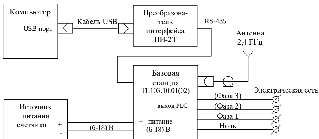
Рисунок Б.1 - Схема подключения базовой станции TE103.10, TE103.10Д к компьютеру и к электрической сети
