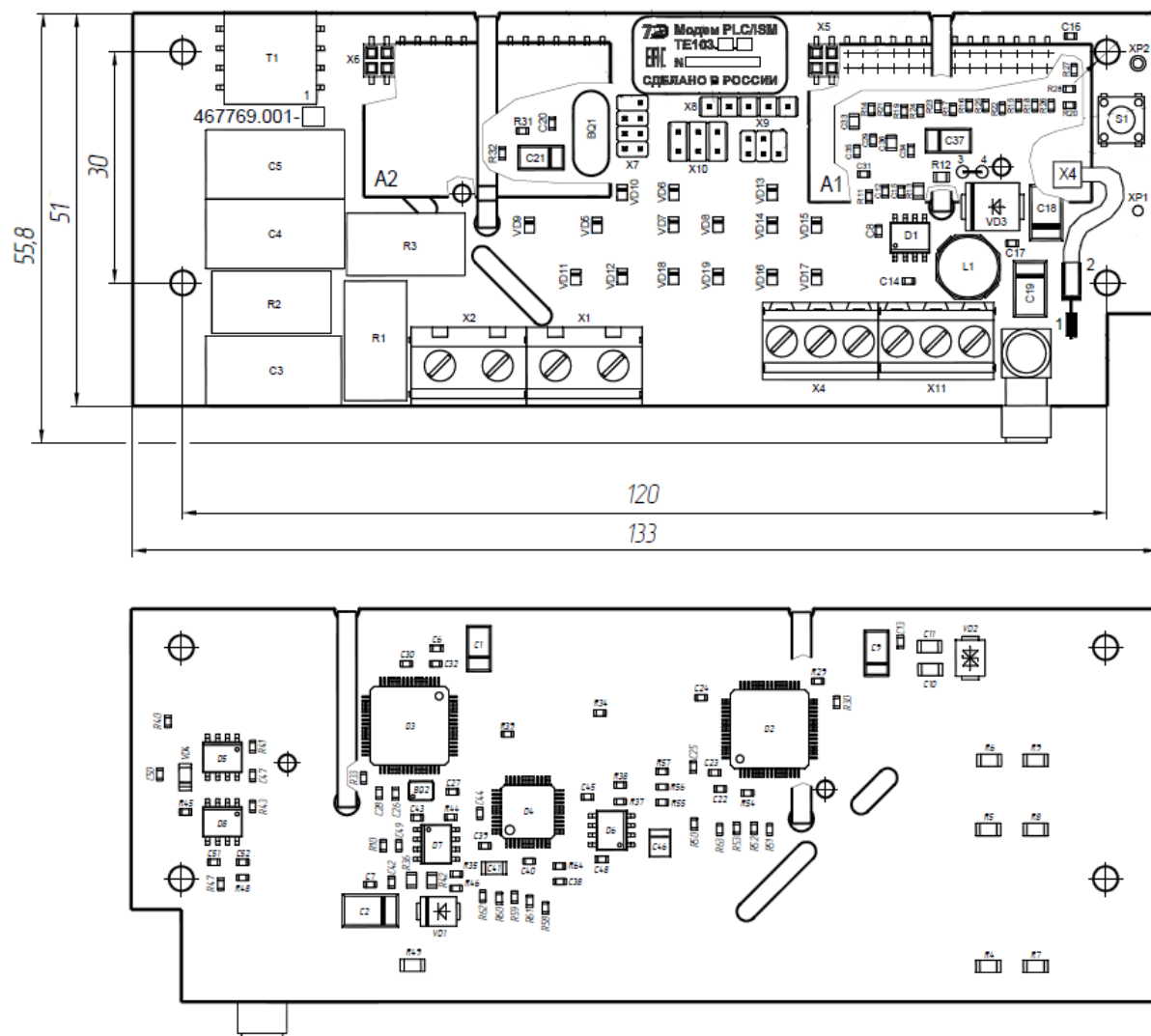
Рисунок А.6 - Габаритный чертеж и установочные размеры модемов TE103.10.01, TE103.10.02
