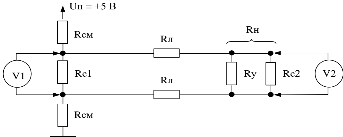
Рисунок Б.2 – Упрощенная эквивалентная схема сети
