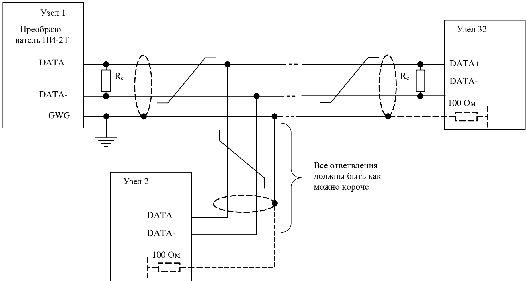
Рисунок Б.4 – Способ соединения приемопередатчиков интерфейса RS-485.
