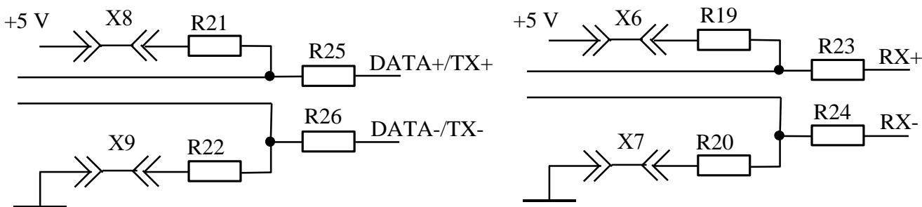
Рисунок 1 - Схема подключения резисторов смещения
