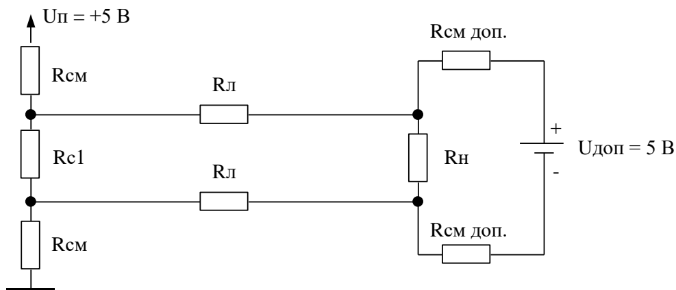
Рисунок Б.3 – Схема подключения дополнительного источника смещения.
